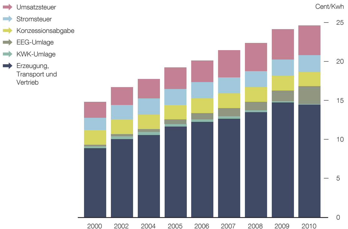
Abbildung 2 Entwicklung der Kostenanteile für eine Kilowattstunde Strom für Haushaltskunden
