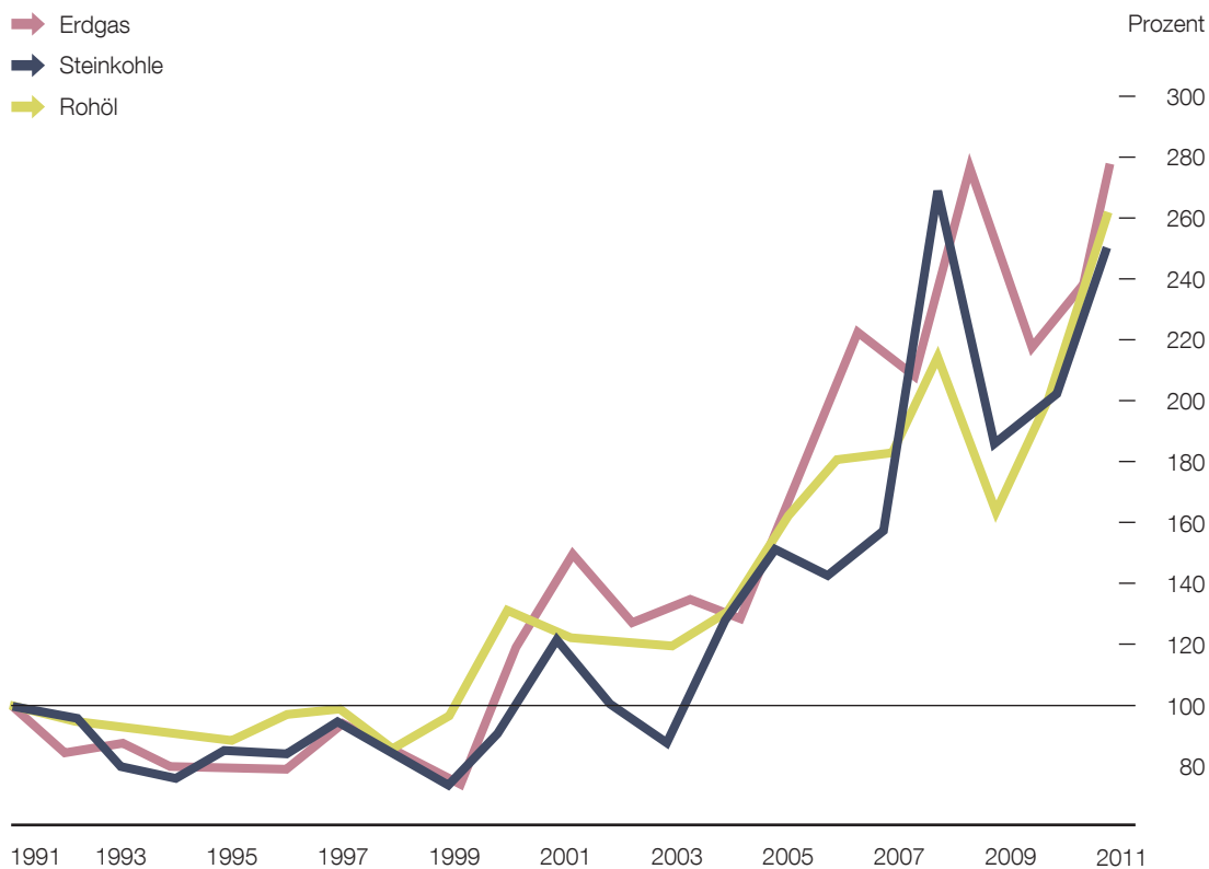
Abbildung 3 Entwicklung der Einfuhrpreise für fossile Energieträger (1991 = 100%)
